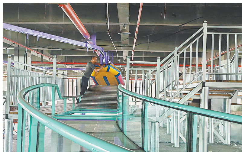
大齐文化旅游集团有限公司工人在调试、安装自动上下船轨道
