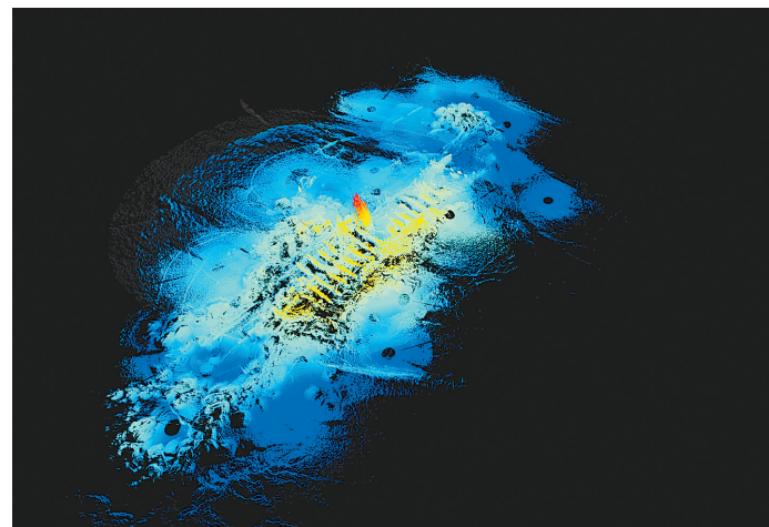
这是2021年“长江口二号”古船多波束声呐扫描合成图。
