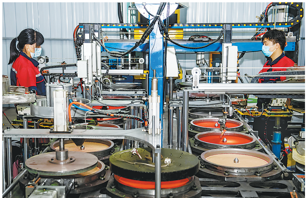
发展高端新材料制造产业 10月12日,工人在河南晟仕博新材料科技公司车间内加工磨具。该公司位于郟县产业集聚区,总投资5亿元,主要从事高端新材料磨具、磨料、船舶辅助配件等的制造。目前,该公司已投资2.78亿元,引进磨料磨具自动化生产设备50台,产品广泛应用于石化、航空、风电等领域,远销北美、欧洲等国际市场。本报记者 王尧 摄
