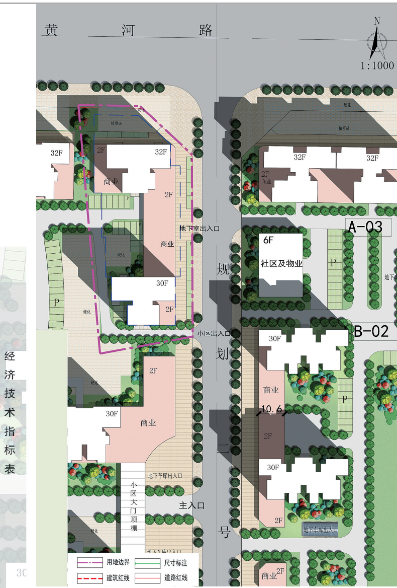
平面图
