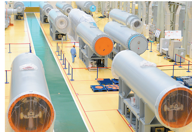
工人在平高集团东区厂房内记录GIS产品信息。近年来，平高集团抓住“关键核心技术开发”和“市场开发”关键环节，建立起了以企业为主体、产学研相结合的自主创新体系，先后参与编制国家、行业标准30余项，并成功跻身全国38家国家高端装备制造标准化试点单位行列。 [本报记者 王尧 摄]
