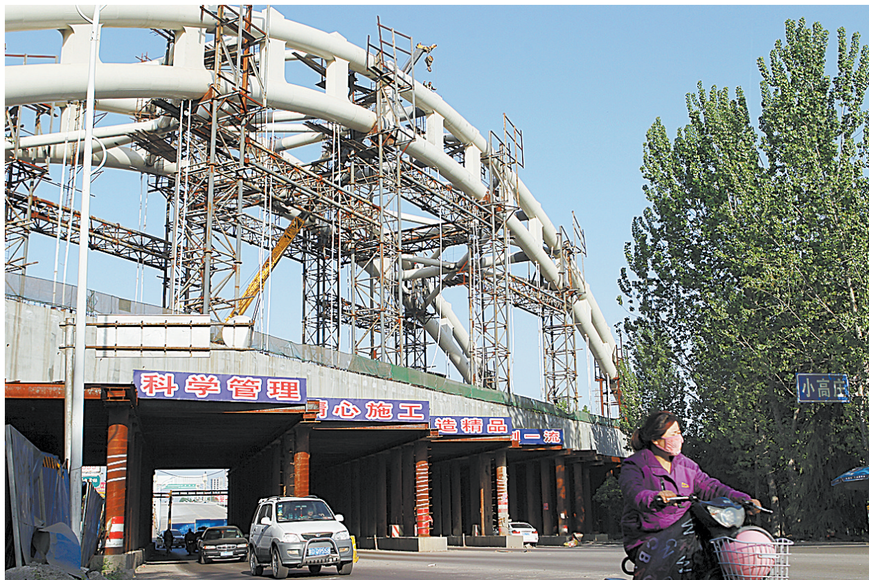
4月13日,工人拆除脚手架。全长1472.66米的孟平铁路复线工程特大桥横跨两条交通干线,建设单位对许南路东侧的跨242省道大桥采
