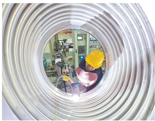
河南平高电力设备有限公司员工在利用自动焊机焊接波纹管
